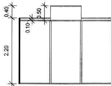
Vista Frontal - Stand Esc.: 1/50
